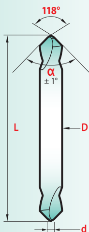
CHANFREIN LONGITUDINAL LONGITUDINAL CHAMFER CHAFLANES LONGITUDINALES SMUSSI LONGITUDINALI
